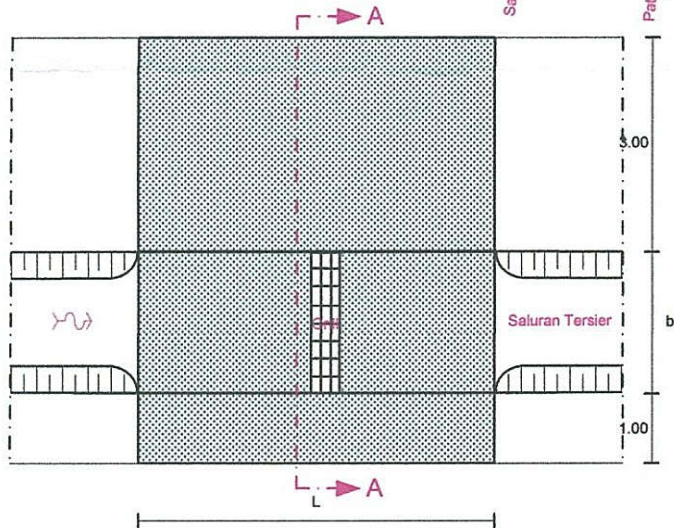
DENAH JEMBATAN H=1:200 V=1:100
