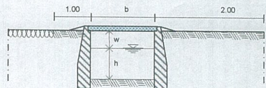
POTONGAN A-A H=1:100 V=1:100
