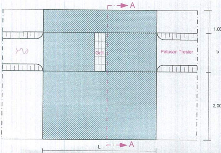
DENAH JEMBATAN H=1:200 V=1:100
