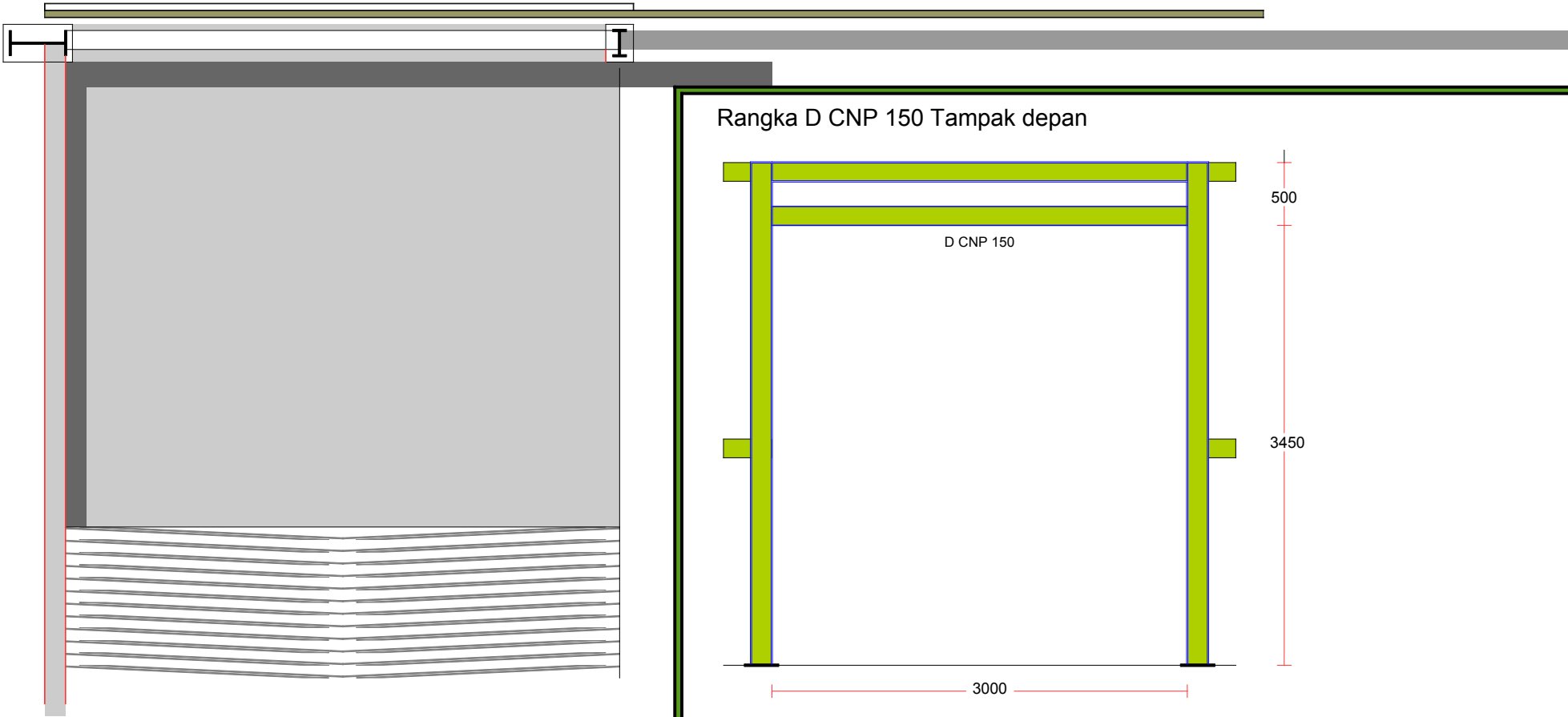
Tampak Atas Existing
